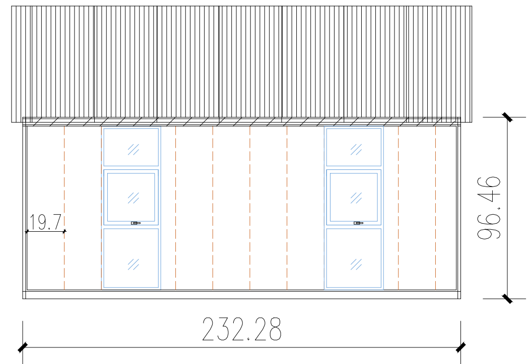
Right elevation
